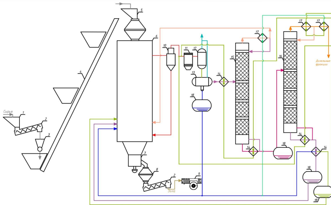
Рисунок 5.13 — Технологическая схема газификации углеводородсодержащих отходов в соответствии с технологией Г19-1
