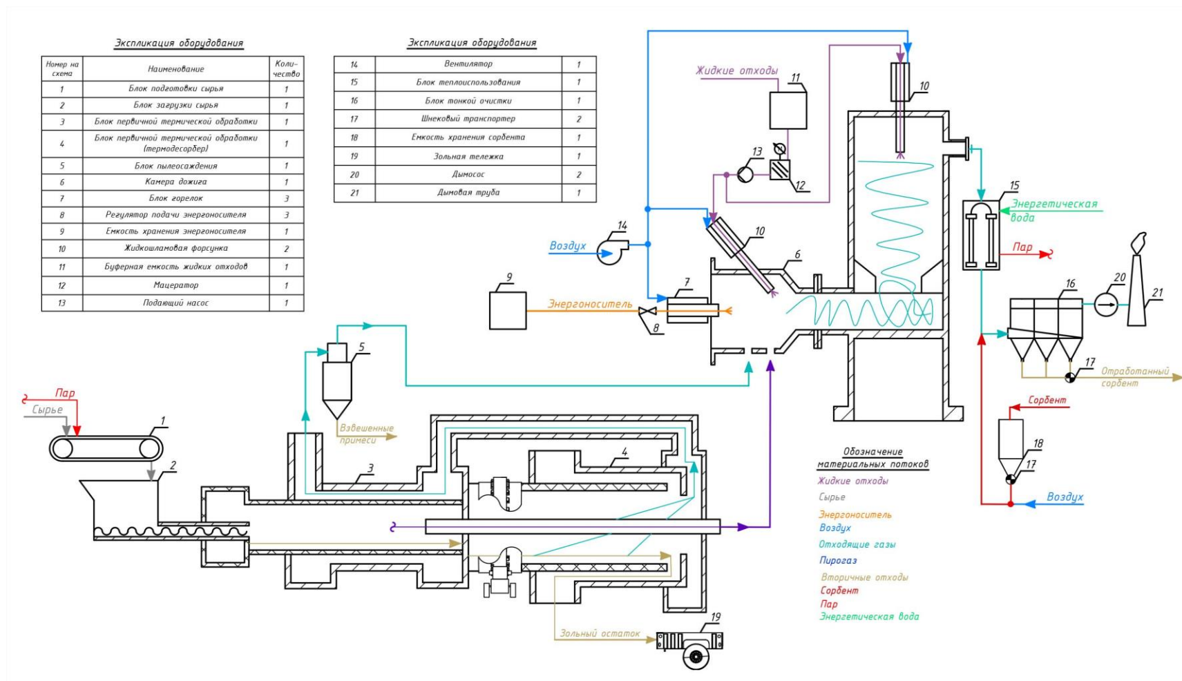
Рисунок 5.14 — Технологическая схема комбинации пиролиза, термодесорбции, сжигания в соответствии с технологией И23-4 (см. таблицу 5.5)
