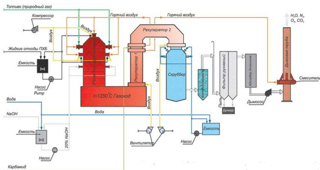
Рисунок 2.24 — Принципиальная технологическая схема установки высокотемпературного обезвреживания жидких ПХБ [39], [40]
