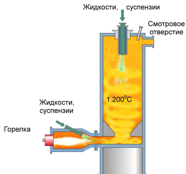
Рисунок 5.19 — Пример конструкции и принципа работы оборудования для высокотурбулентного сжигания отходов и дожига пирогозов (П23) (см. таблицу 5.5)
