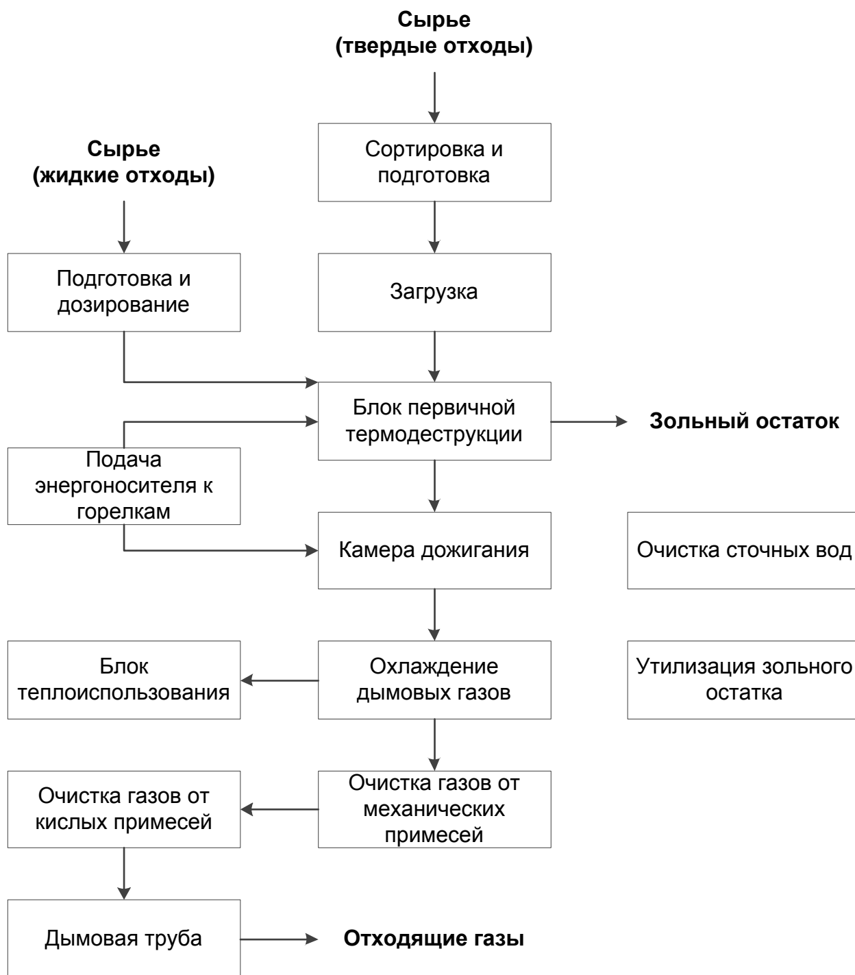
Рисунок 5.1 — Общая схема сжигания отходов
