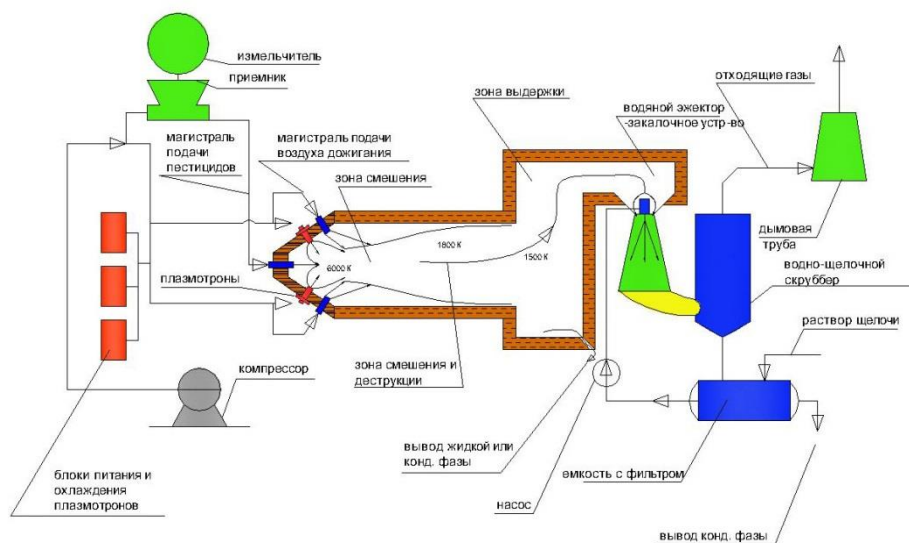
Рисунок 2.13 — Технологическая схема установки для плазменной переработки пестицидов [23]
