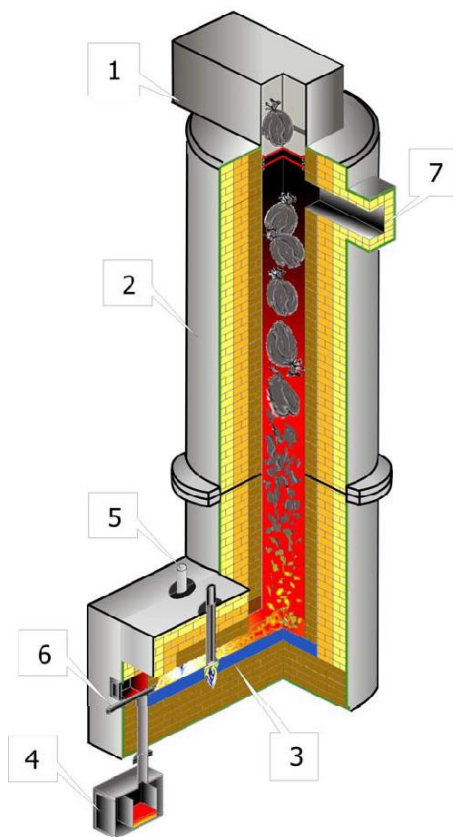
1 — узел загрузки; 2 — шахта; 3 — под; 4 — бокс приема шлака; 5 — плазматрон; 6 — стопор; 7 — выход пирогаза
