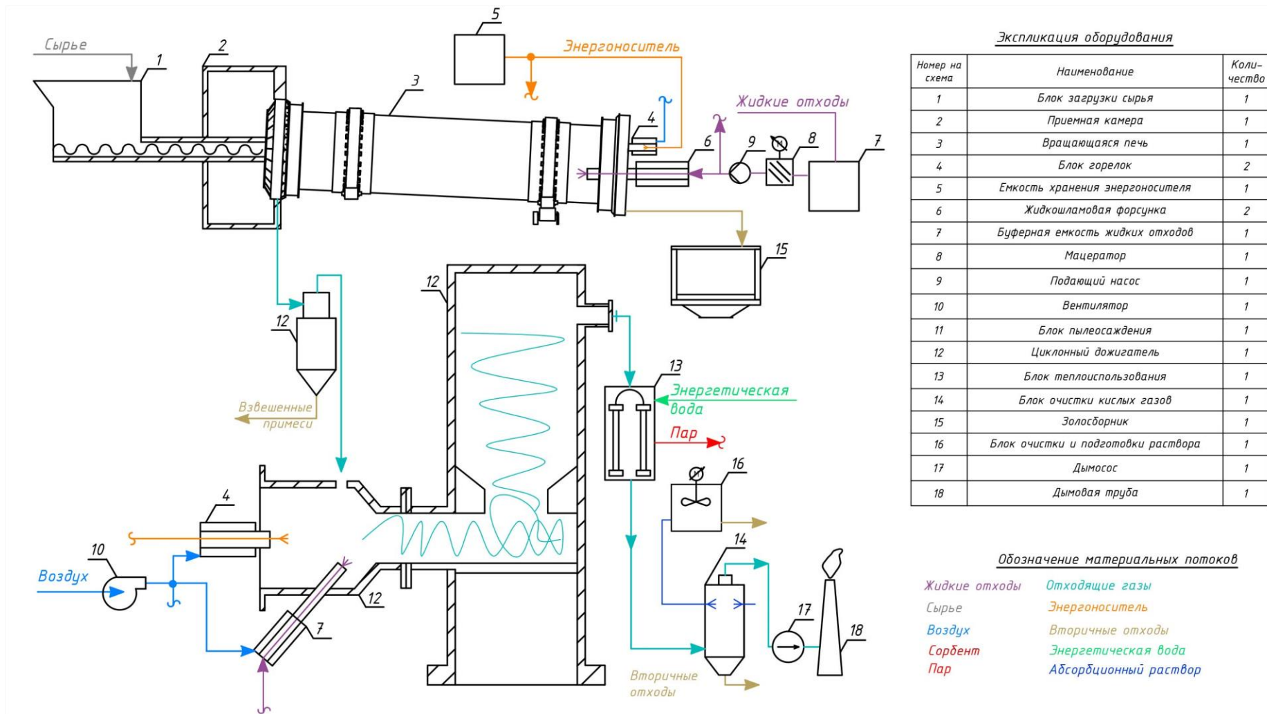
Рисунок 5.12 — Технологическая схема высокотемпературного пиролиза в соответствии с технологией П23-3В
