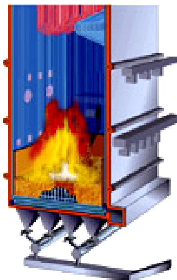
Рисунок 2.10 — Топка с кипящим слоем [11]
