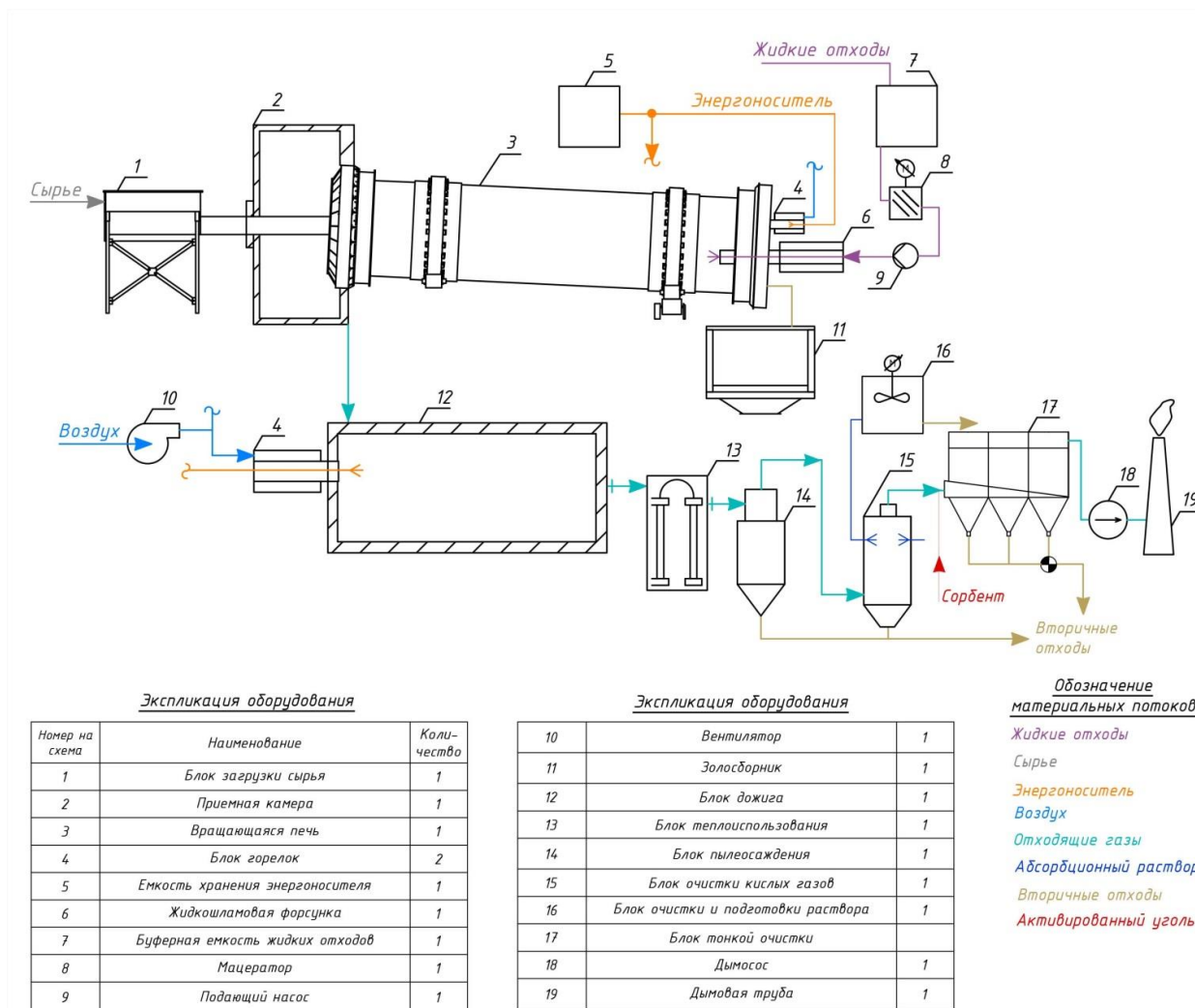
Рисунок 5.7 — Принципиальная технологическая схема сжигания отходов во вращающейся барабанной печи на базе технологических решений С2-4В, С5-1В, С6-1В, С14-1В, С14-2В, С15-3В (см. таблицу 5.5)
