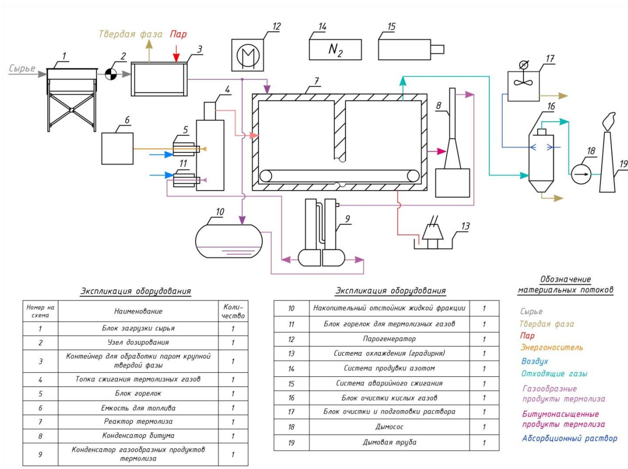
Рисунок 5.11 — Технологическая схема термолитной переработки нефтешламов в соответствии с технологией П4-1 (см. таблицу 5.5)
