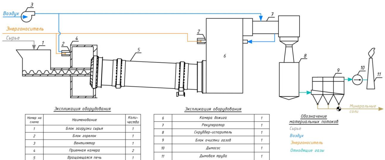
Рисунок 5.17 — Технологическая схема огневого обезвреживания пришедших в негодность пестицидов
