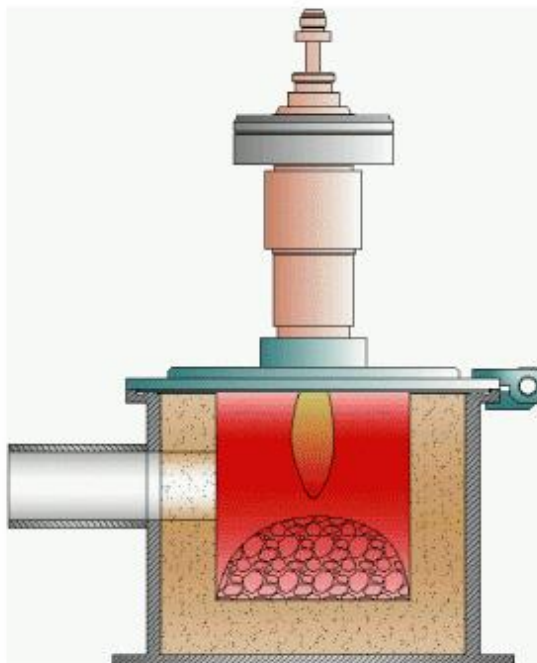
Рисунок 2.17 — Плазменная печь для обезвреживания медико-биологических отходов [27]
