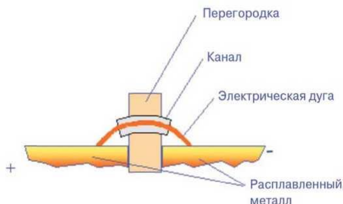
Рисунок 7.1 — Схема плазмотрона с жидкометаллическими электродами [78]
