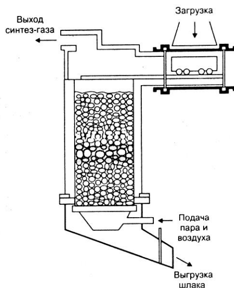
Рисунок 2.6 — Шахтная печь [19]
